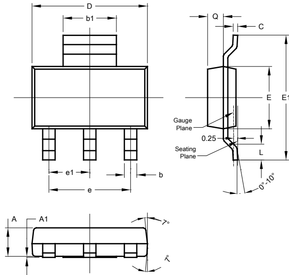
SOT223
